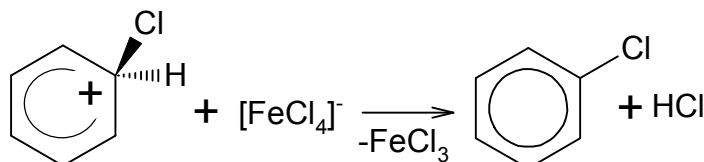
chlorbenzen
