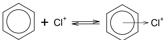
\pi -komplex
