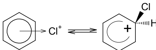
\sigma -komplex
